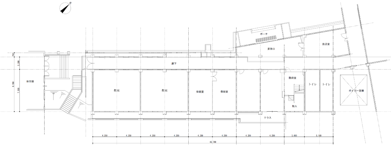
普通教室棟1階
