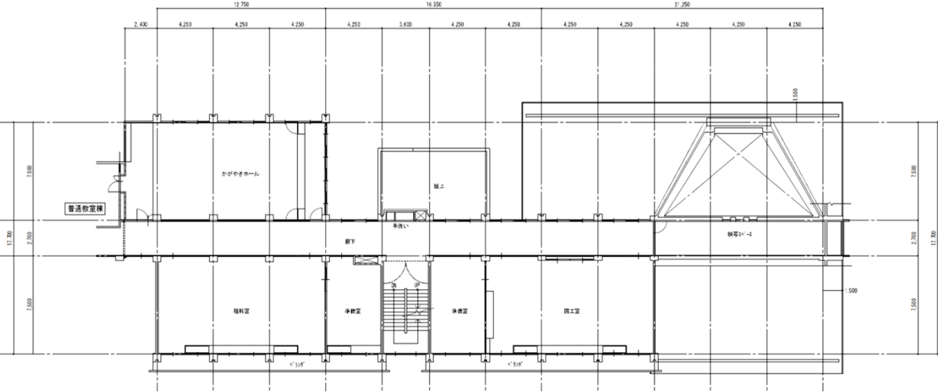
特別教室棟2階
