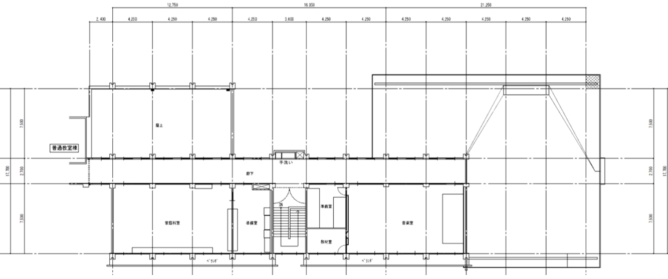
特別教室棟3階
