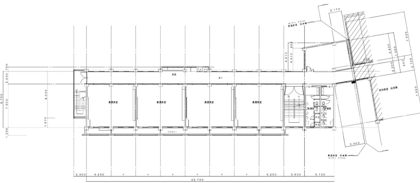
普通教室棟3階
