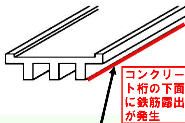
主桁の損傷（鉄筋露出）
